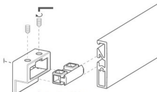
> Assemblage de la barre de fond de hotte
